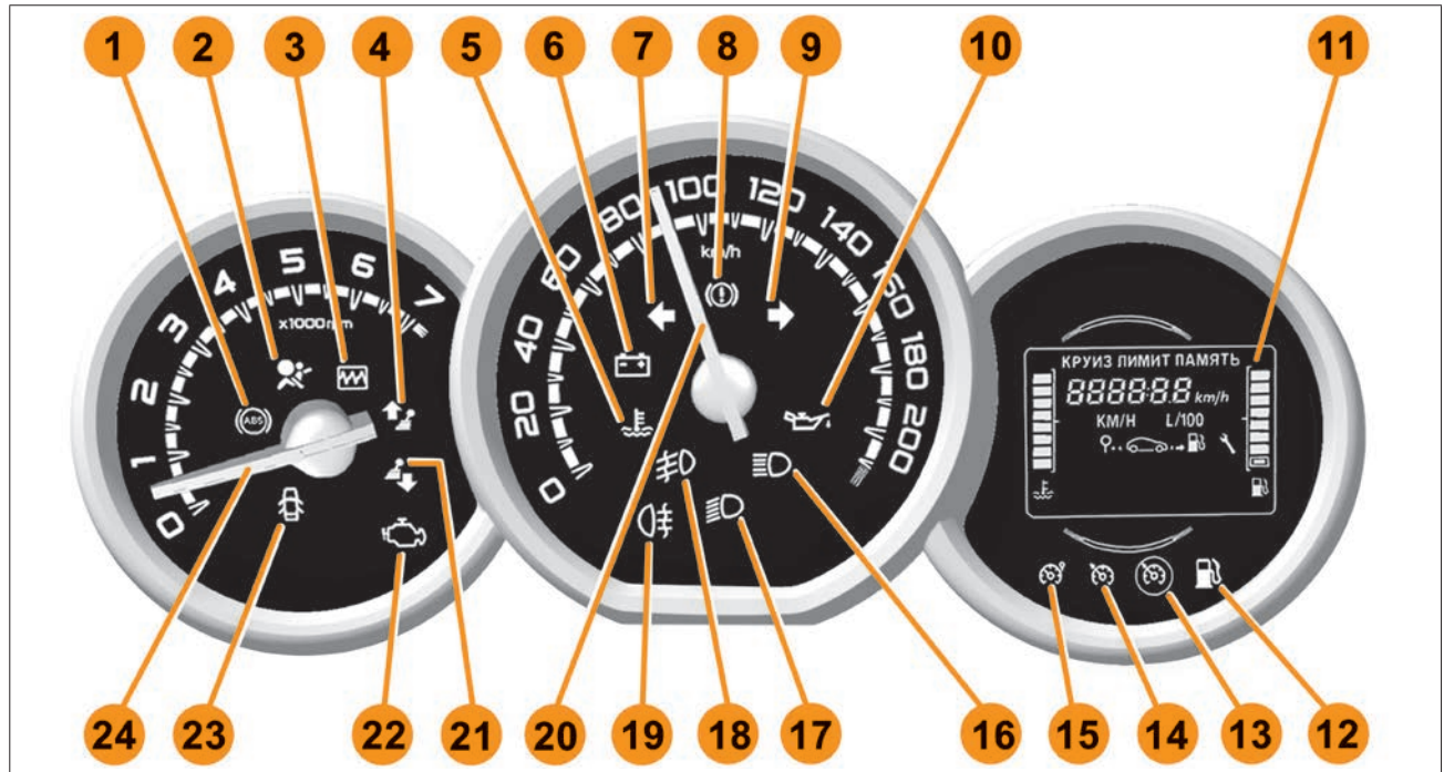
Рис. 3.2.1. Комбинация приборов (в варианном исполнении)
