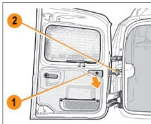
Рис. 1.4.6. Полное открытие большой двери багажного отделения
