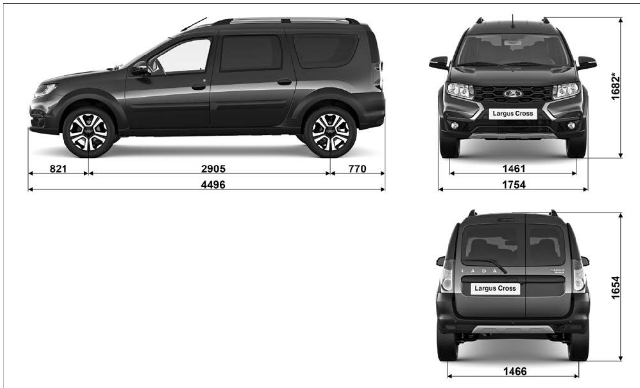
Рис. 7.2.3. Габаритные (справочные) размеры автомобиля Largus Cross (в варианном исполнении)
