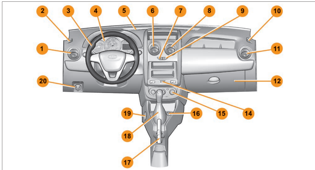
Рис. 3.1.1. Панель приборов в исполнении «Стандарт» (в варианном исполнении)
