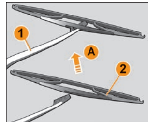
Рис. 6.8.3. Замена щетки стеклоочистителя заднего стекла (в варианном исполнении)
