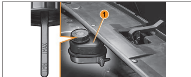
Рис. 6.7.1. Бачок гидроусилителя рулевого управления (в варианном исполнении)
