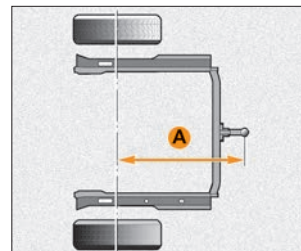
Рис. 5.15.1. Схема размещения ТСУ (в варианном исполнении)
