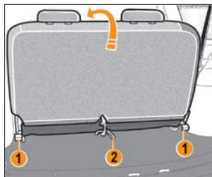
Рис. 2.3.2. Складывание сиденья третьего ряда (в варианном исполнении)
