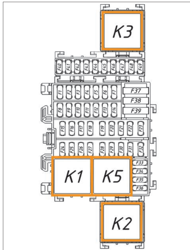
Рис. 8.4.1. Схема расположения предохранителей и реле в монтажном блоке салона (в варианном исполнении)
