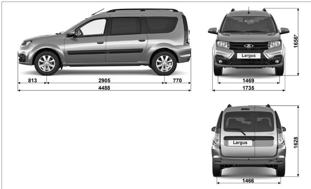
Рис. 7.2.1. Габаритные (справочные) размеры автомобиля L Largus «универсал» (в варианном исполнении)
