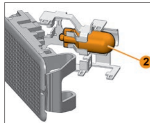
Рис. 6.13.12. Лампа освещения вещевого ящика (в варианном исполнении)
