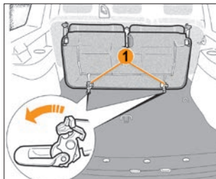
Рис. 2.3.5. Защелки крепления сиденья третьего ряда
