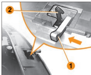
Рис. 6.2.2. Предохранительный крюк замка капота
